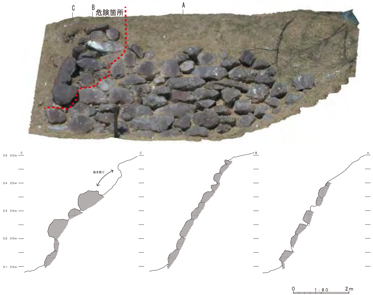
第 6-11 図 伝天守台石垣東部現況図
