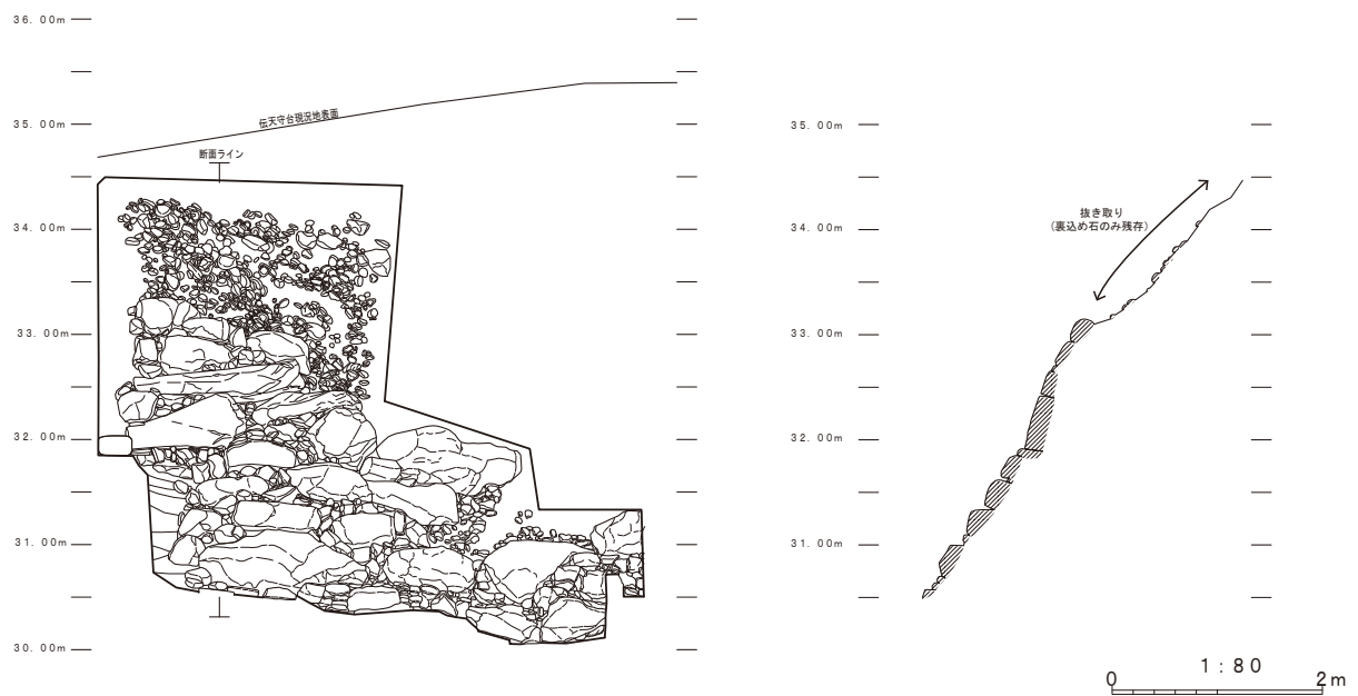
第 6-11 図 伝天守台石垣東部現況図
