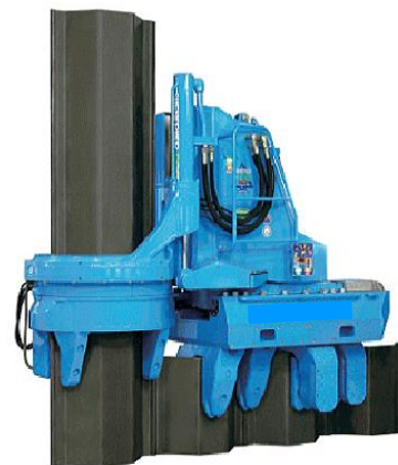
油圧式矢板圧入引抜機
