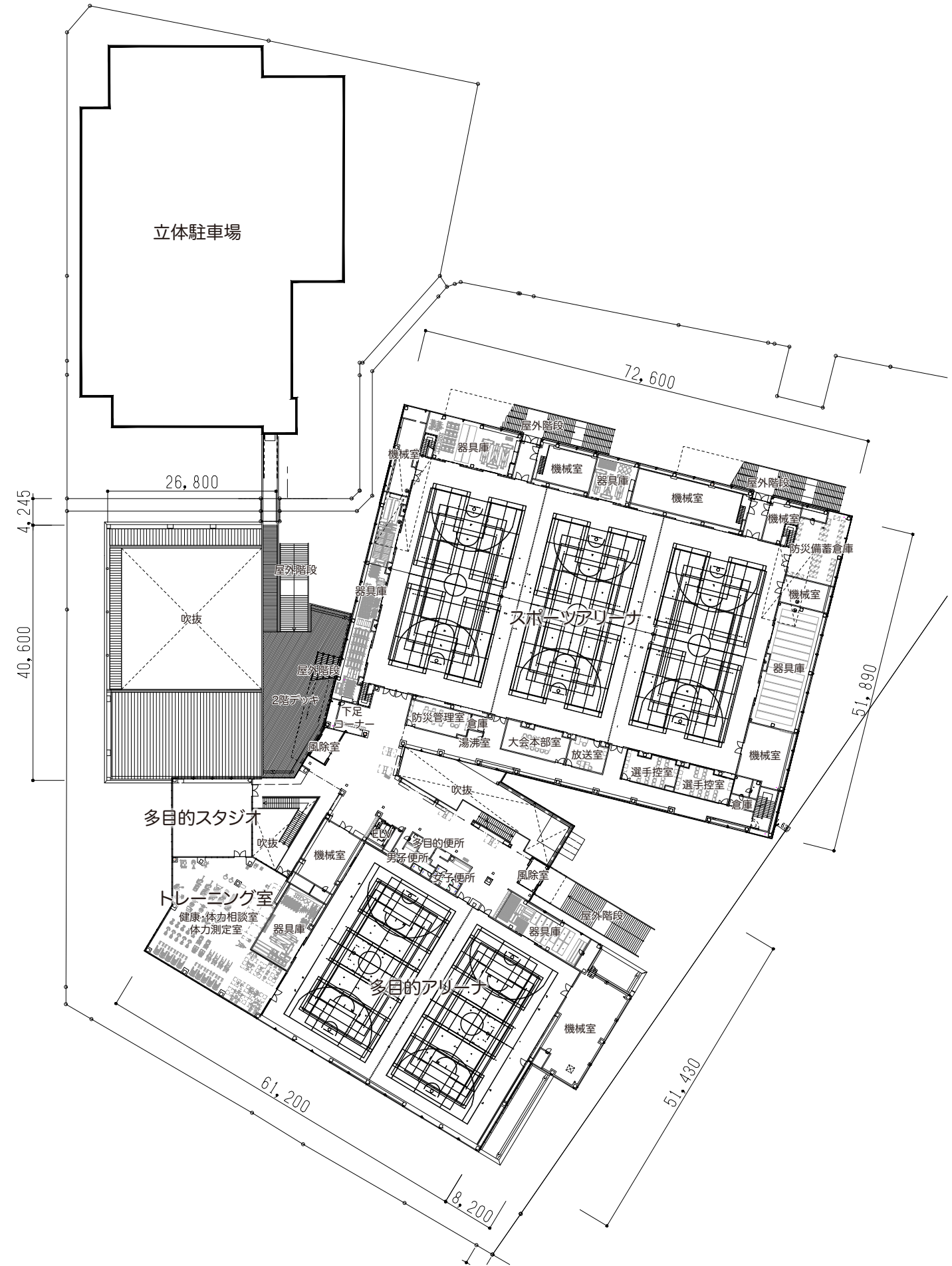
2階平面図
