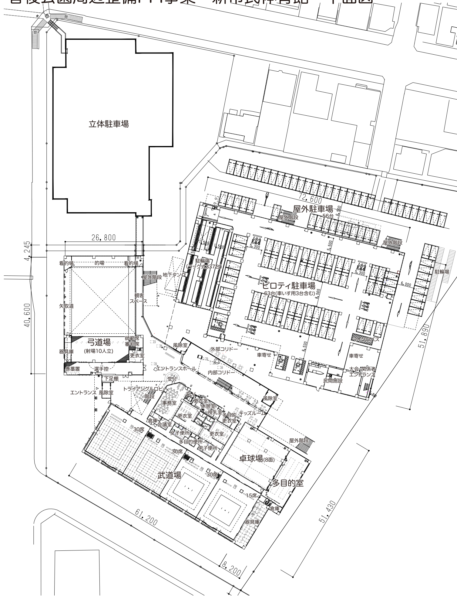
1階平面図
