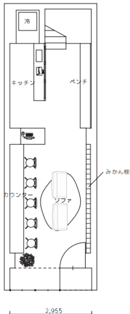
1 階平面図
