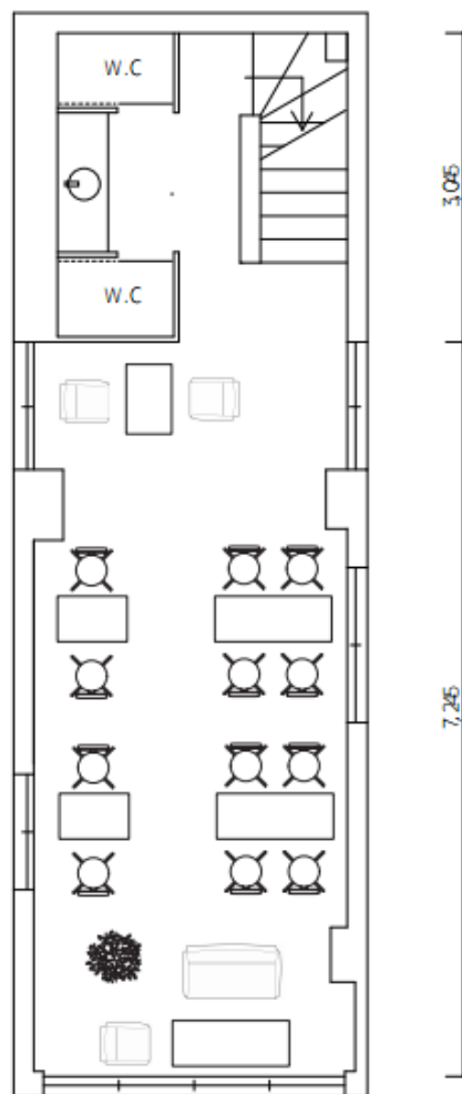
2 階平面図
