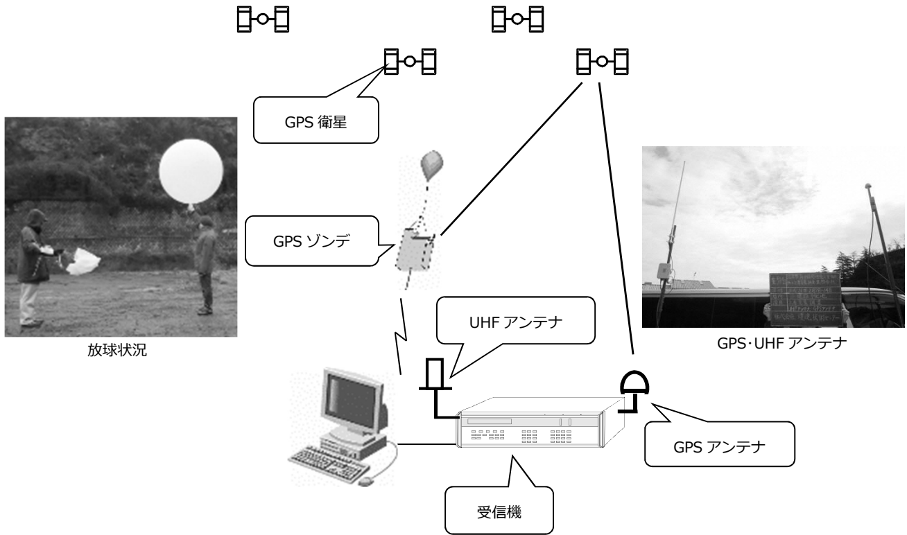
図 1.3 上層気象観測システム
