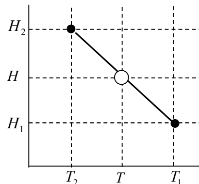
図 1 気温データの内挿処理
