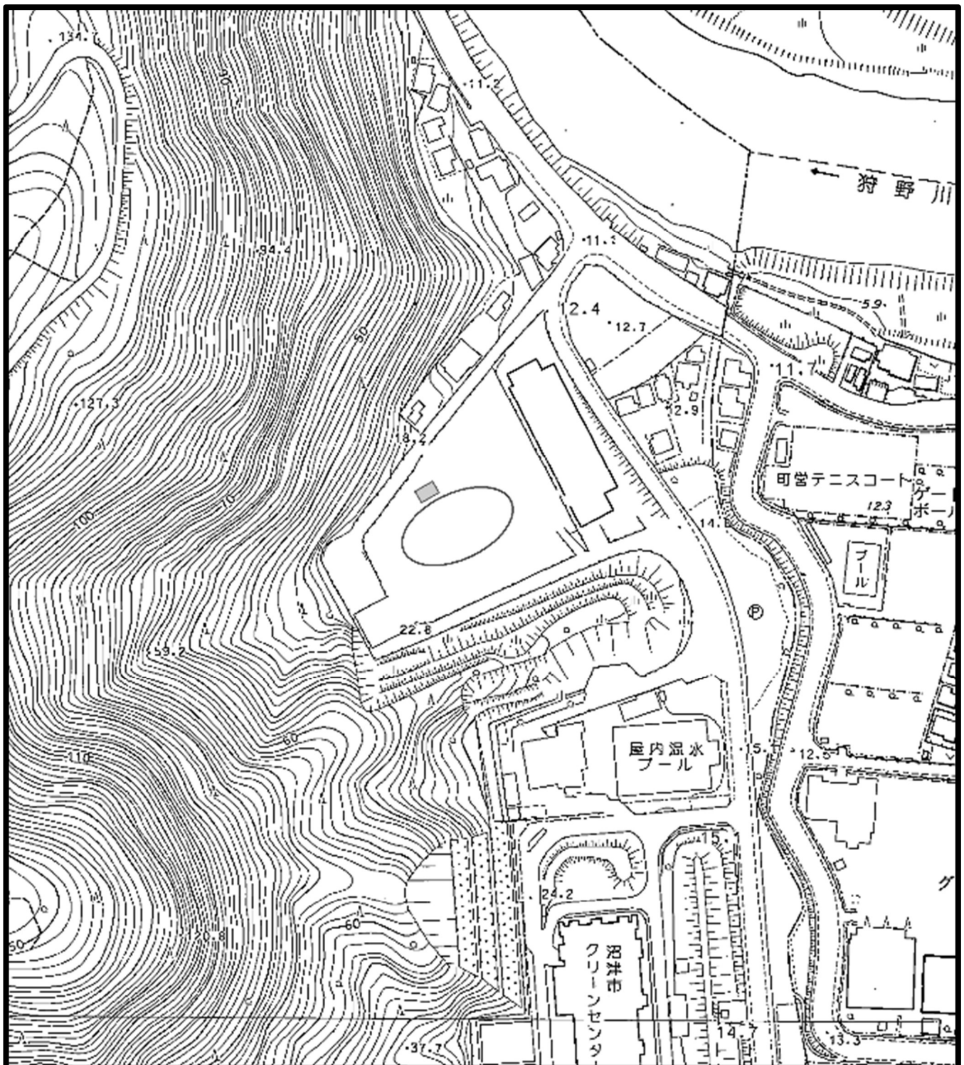
図 1.2.2 観測実施地点位置図 (詳細)
