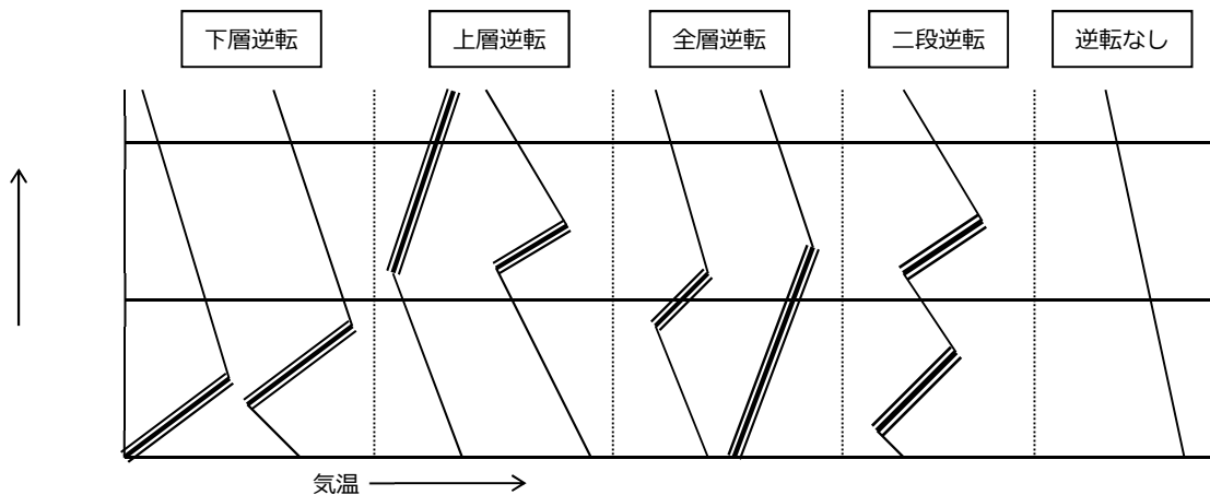
図 2.4.1 逆転層の区分(指定高度 100m の場合)
