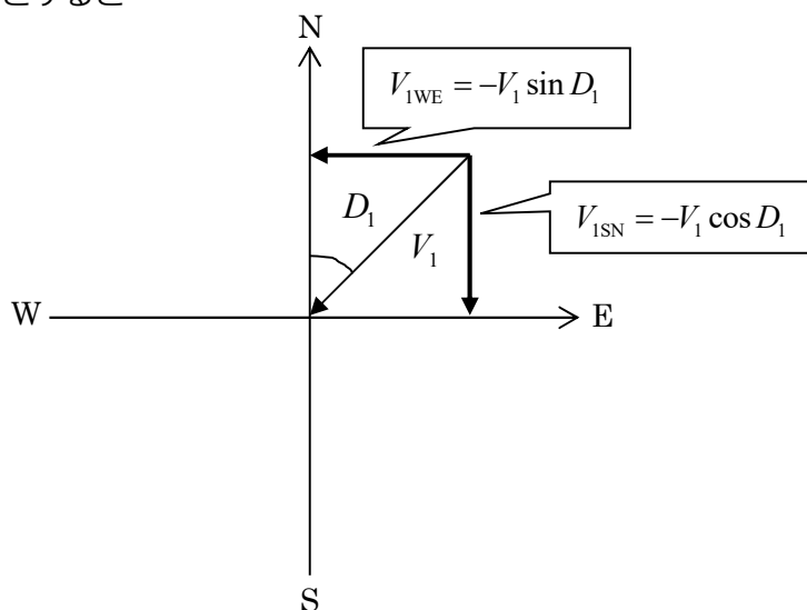
図3 風の成分値の算出
