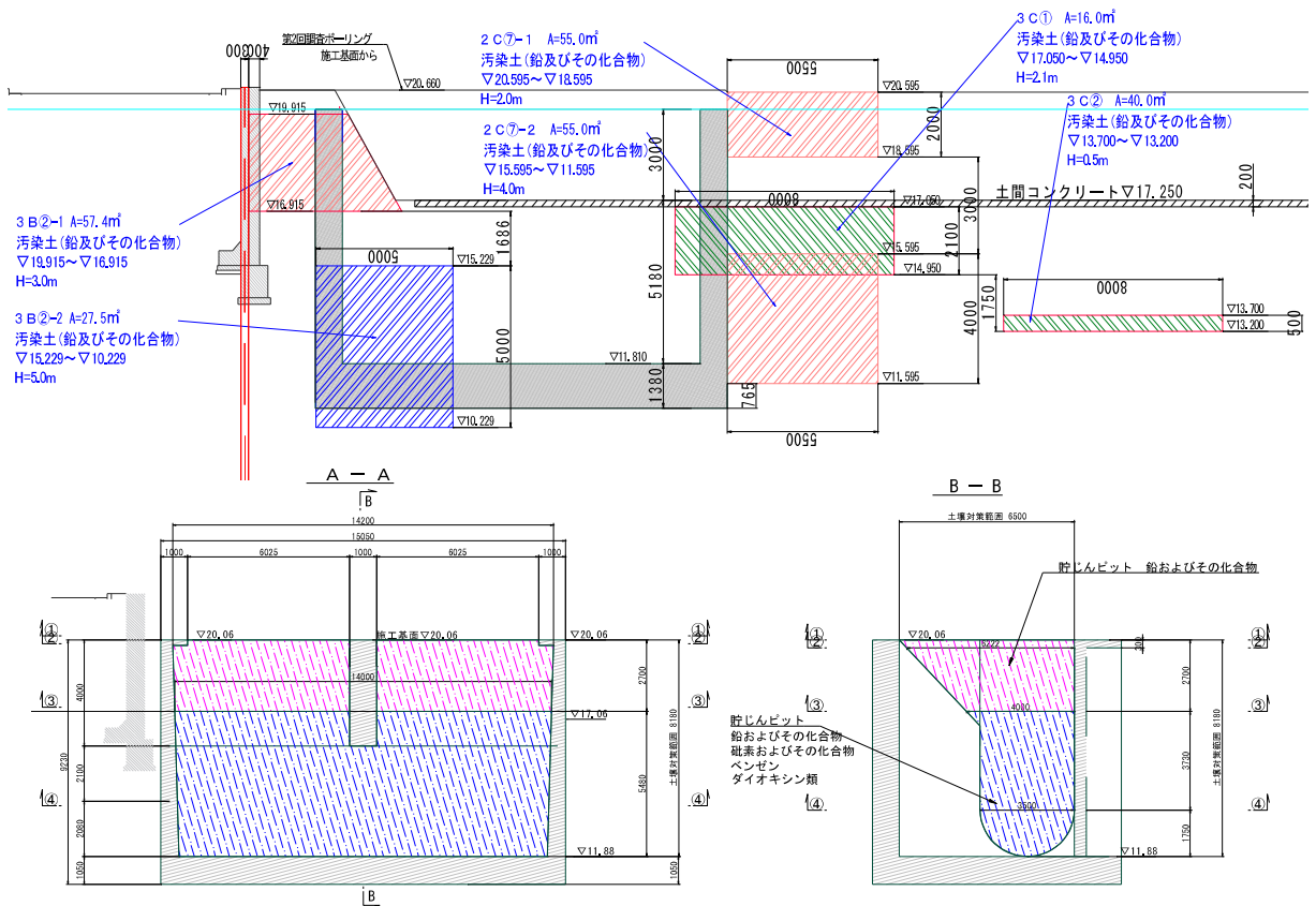
図2. 調査結果(重ね断面図)
