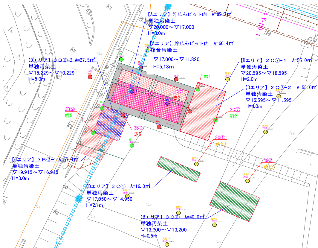
図1. 調査結果(平面図)
