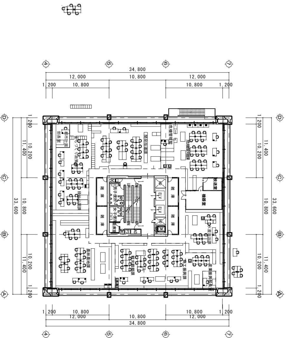
5階平面図 S=1/300
