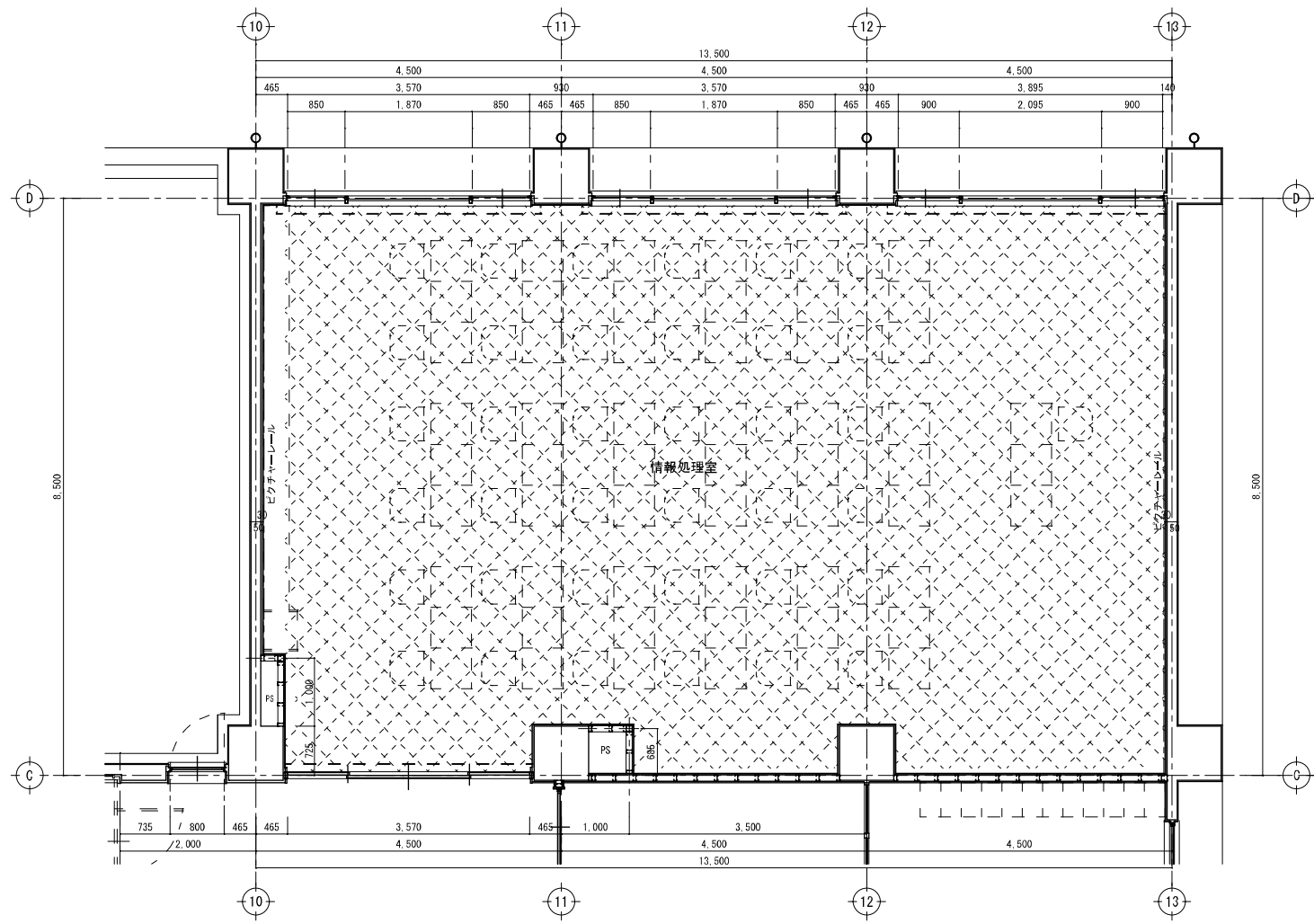
情報処理室平面詳細図 Scale 1:50
