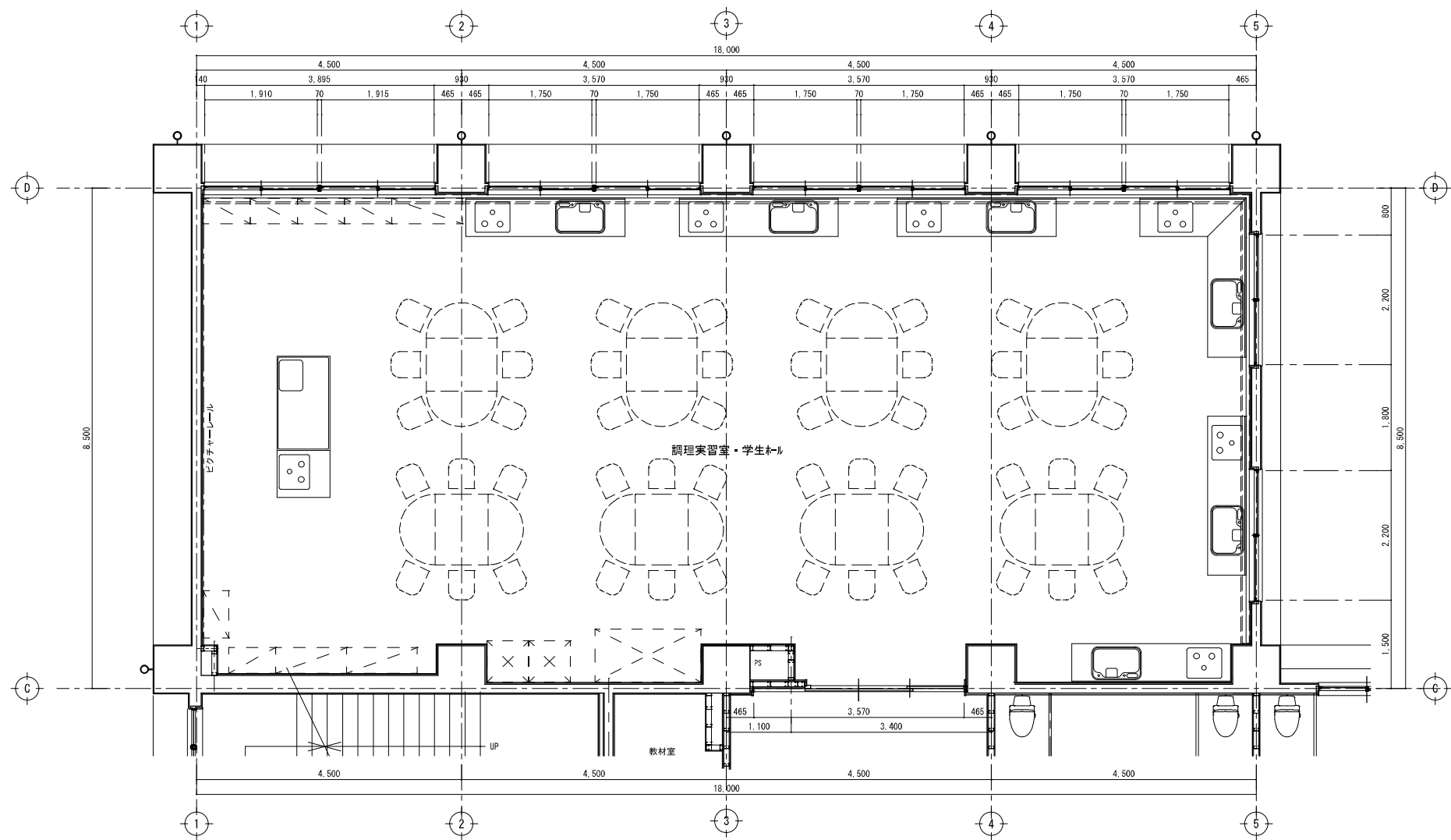
調理実習室・学生ホール平面詳細図 Scale 1 : 50
