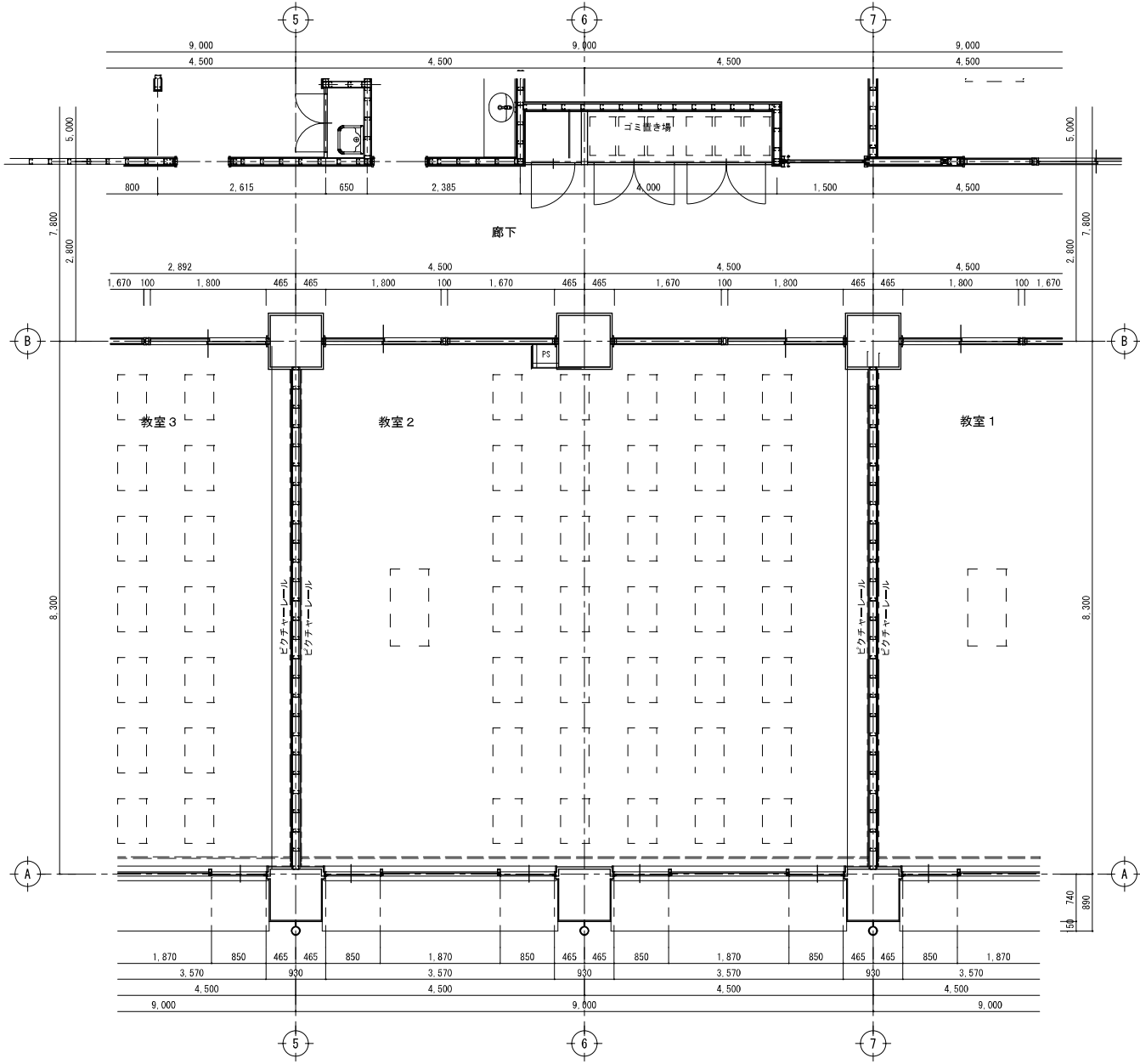
普通教室平面詳細図 Scale 1:50
