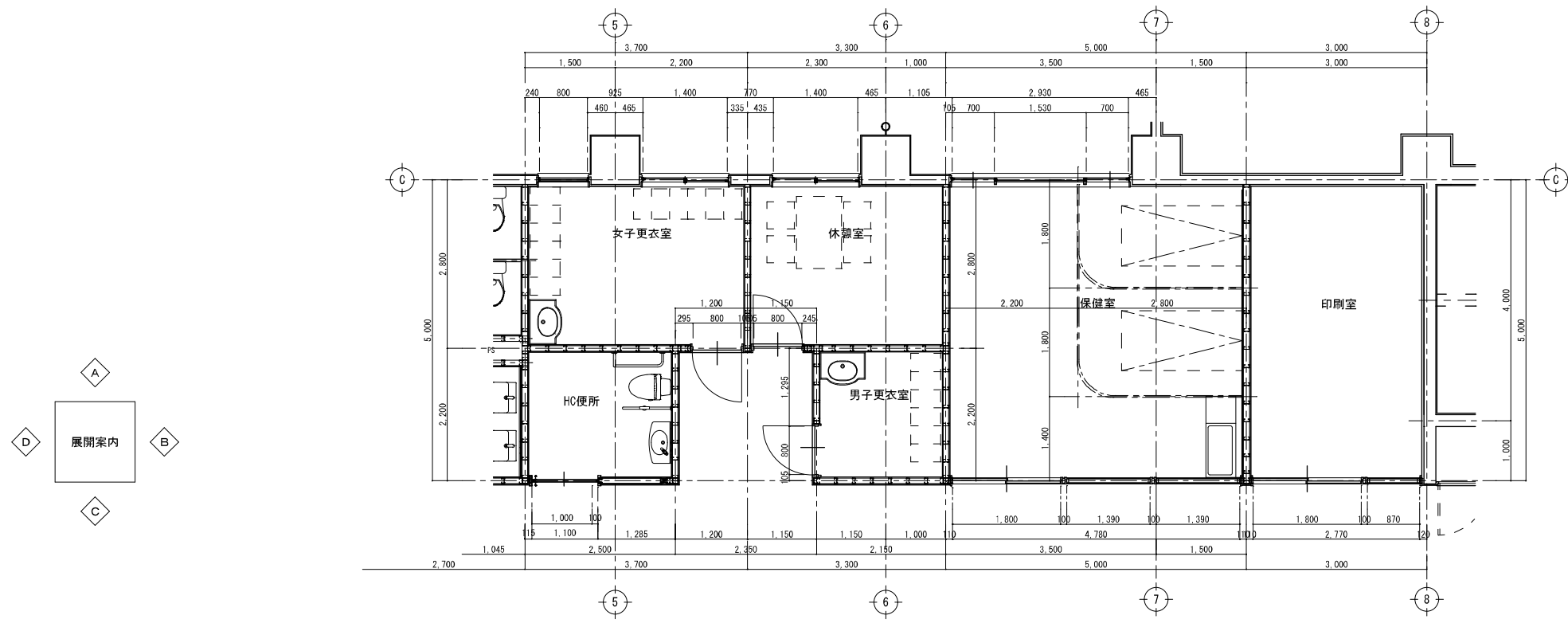
HC便所・男女職員更衣・休憩室・保健室平面詳細図 Scale 1:50
