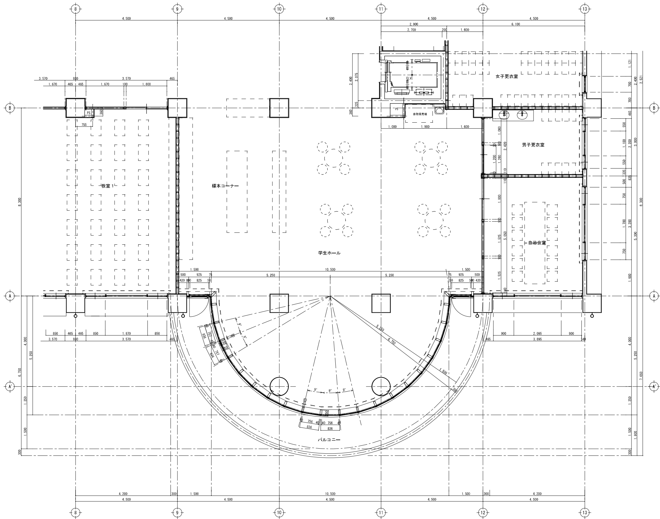
学生ホール・自治会室平面詳細図 Scale 1:50
