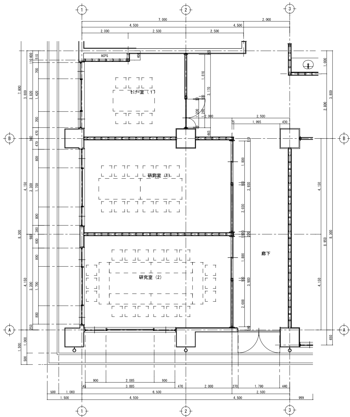
セミナー室・研究室 1・2 平面詳細図 Scale 1:50
