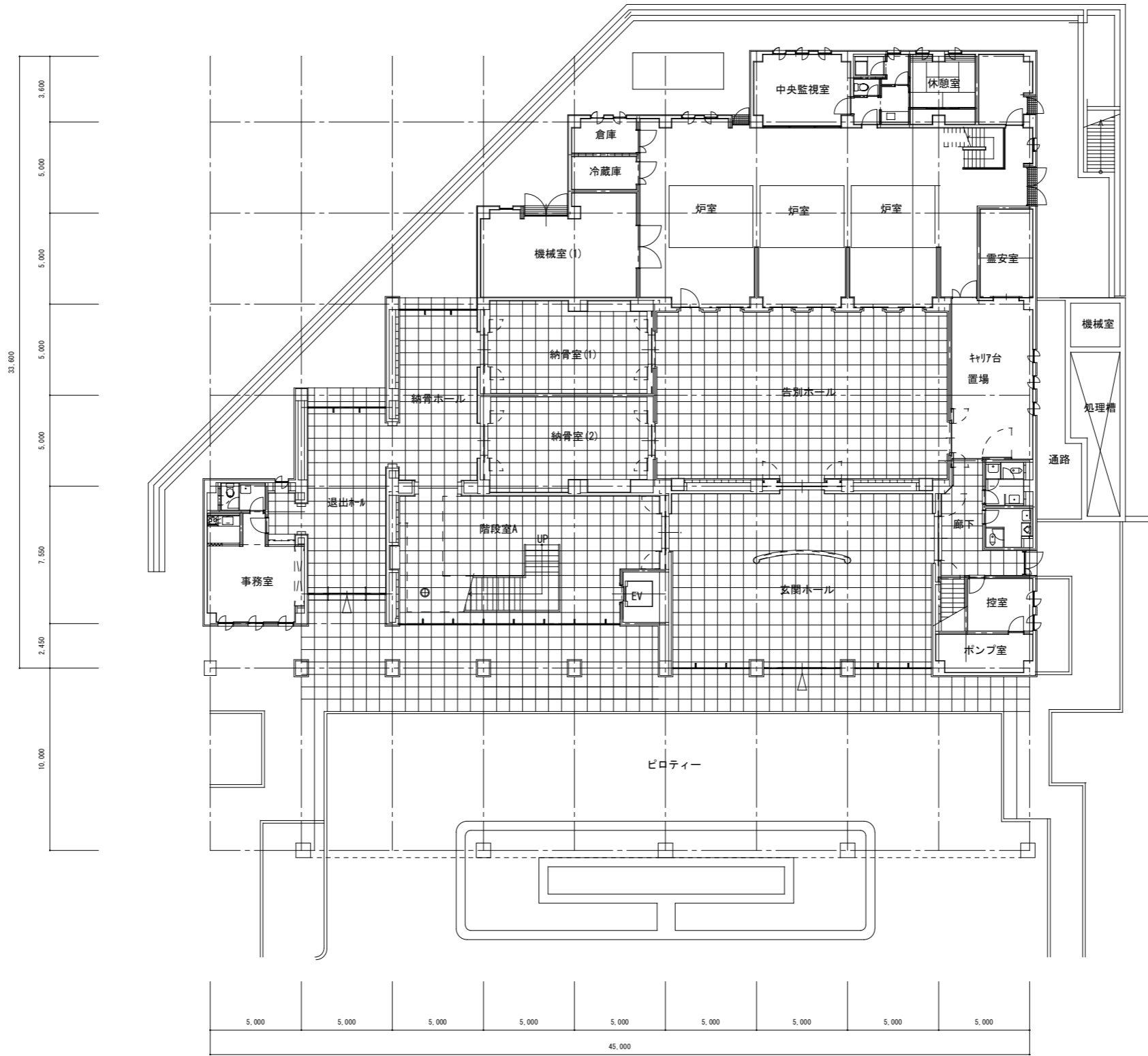
1階 平面図
