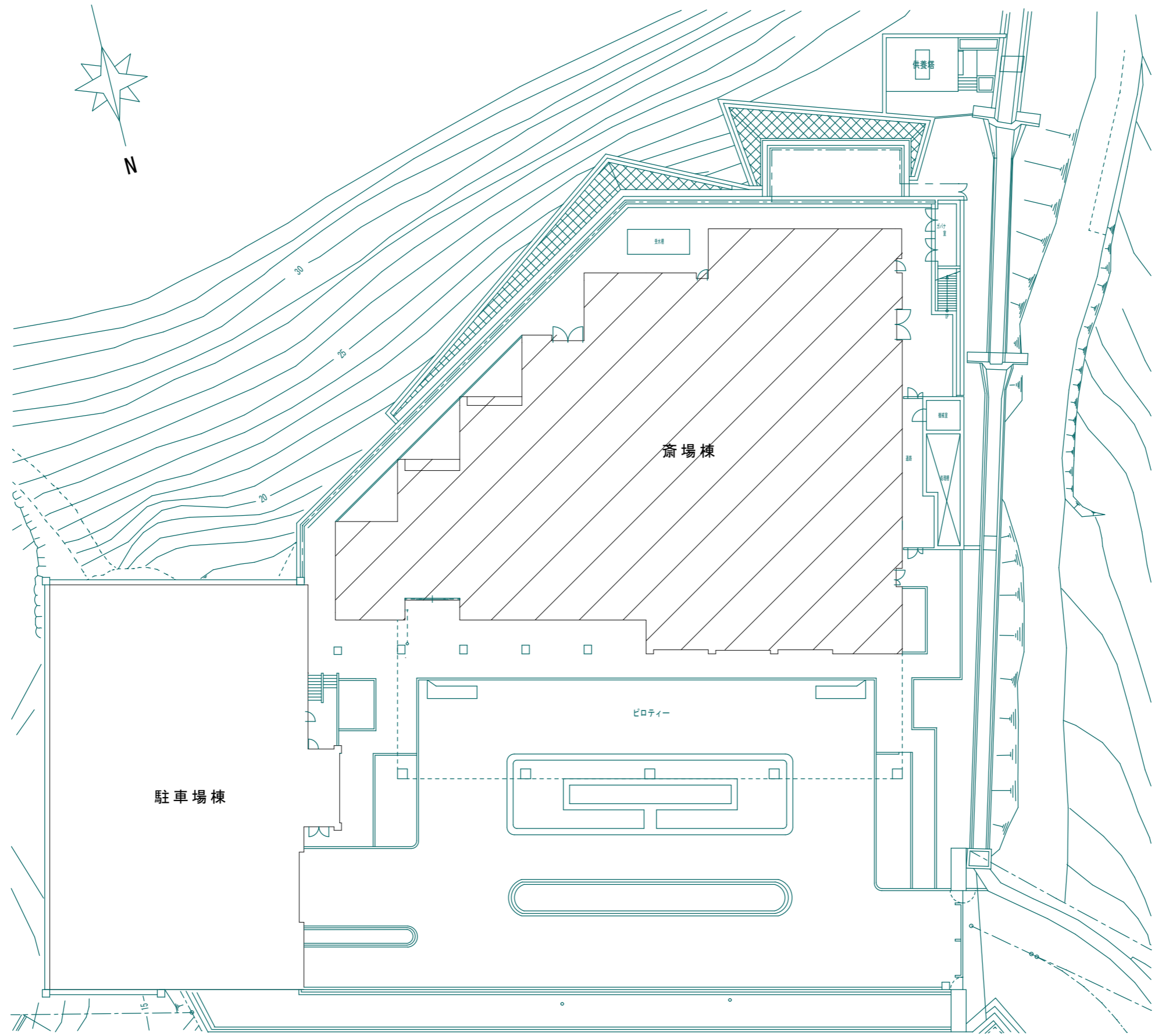
配置図 S=1/100
