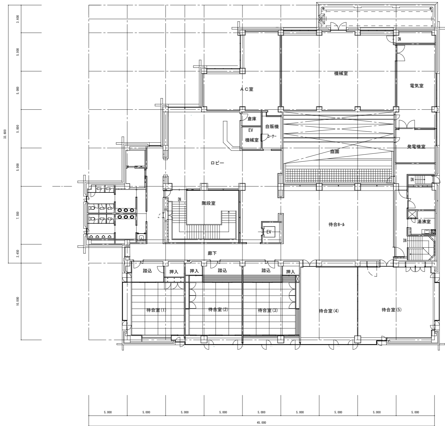
2階 平面図
