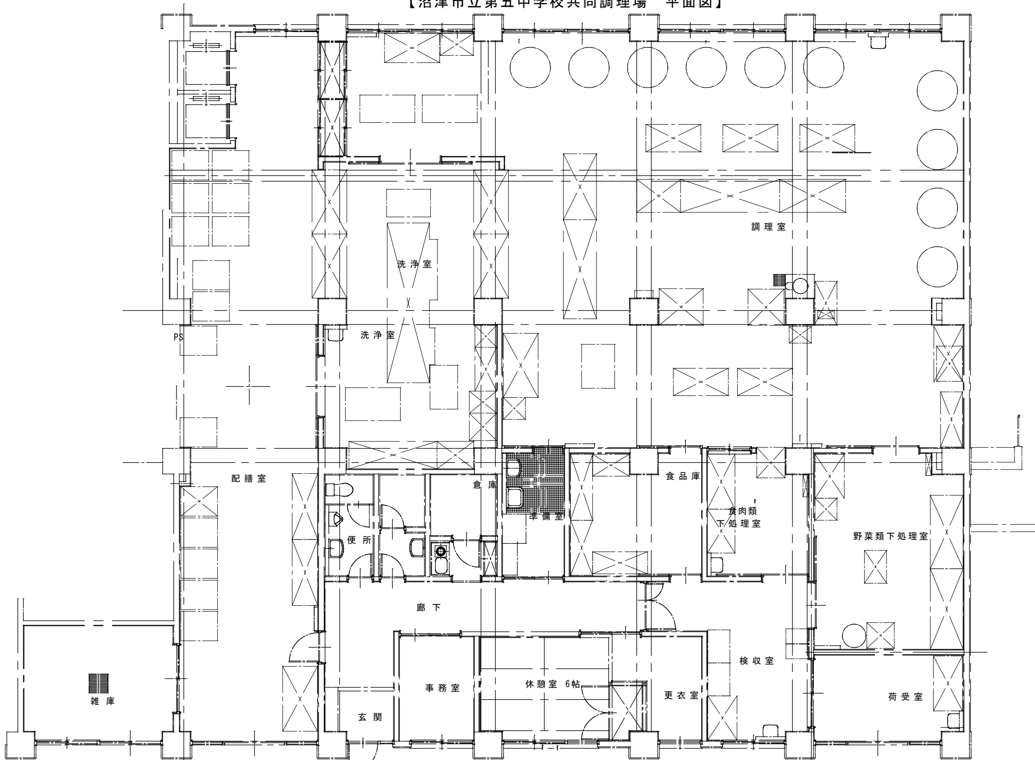
【沼津市立第五中学校共同調理場 平面図】
