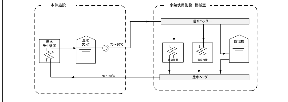
図2-5 外部熱供給条件
