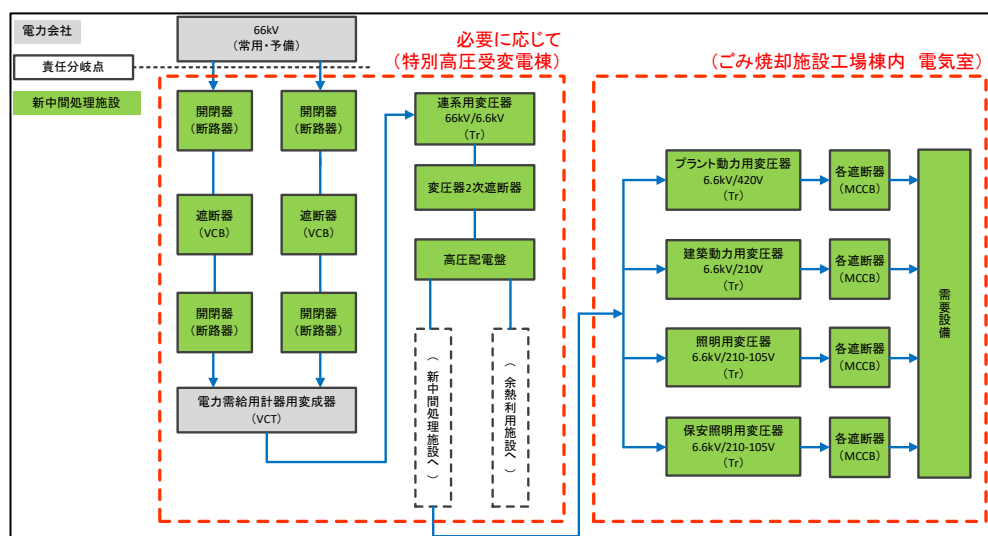
図2-1 電力受変電系統図（参考）
