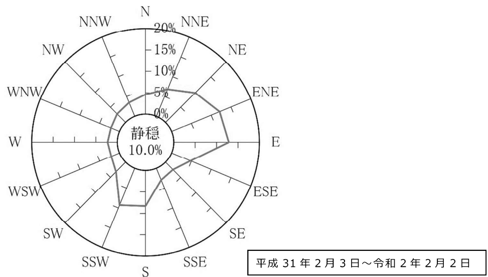
図 3.1.10 外原固定局の風配図
