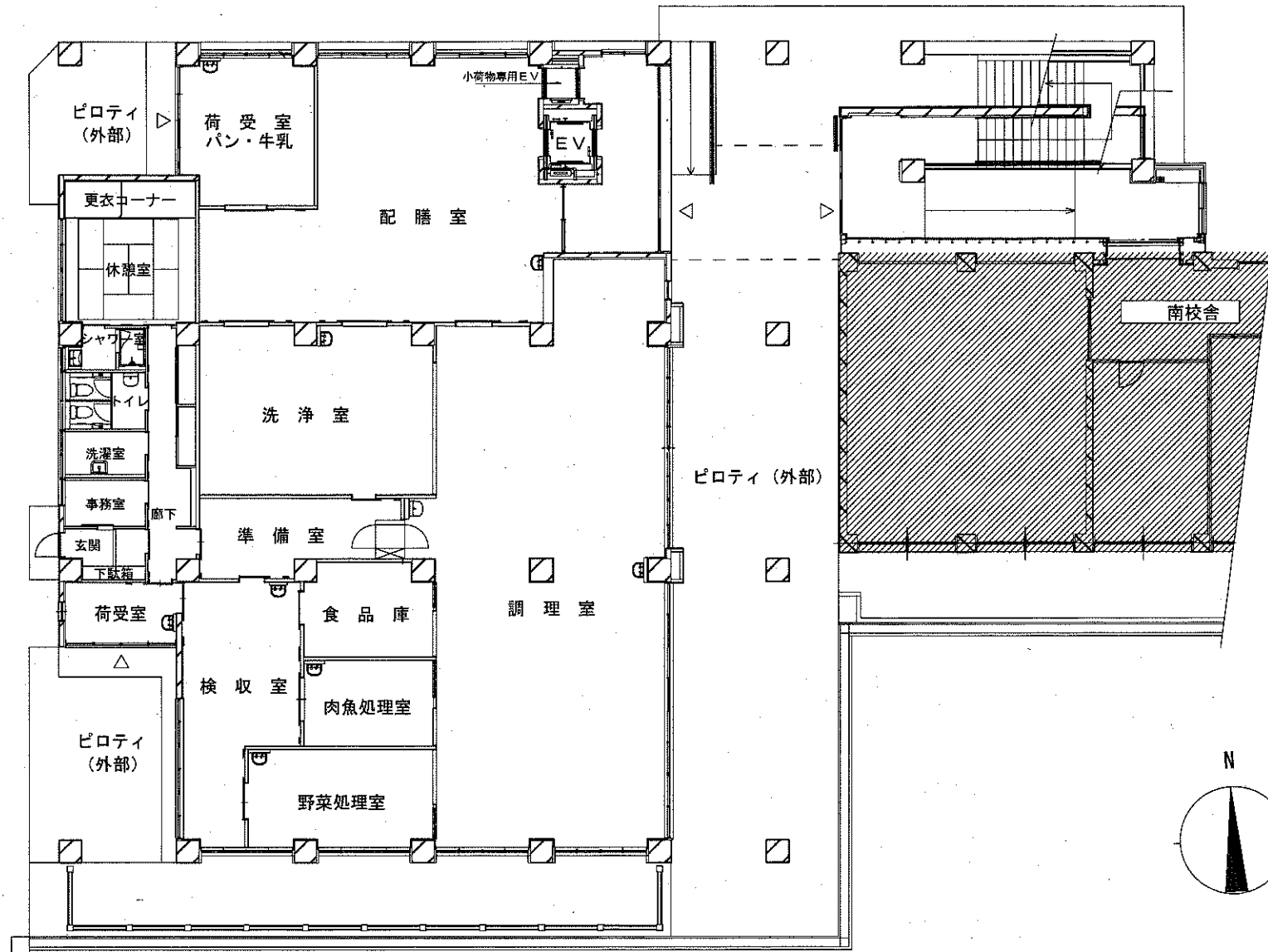
【沼津市立門池小学校共同調理場 平面図】
